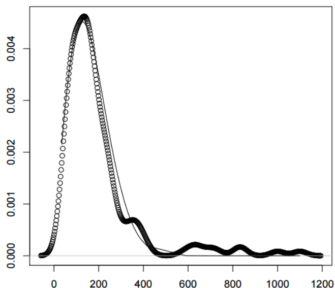
Рисунок 1 – Плотность распределения количества ретвитов, полученных из реальной сети (аппроксимация распределением Вейбулла при k = 1.9 , \lambda = 180 )
