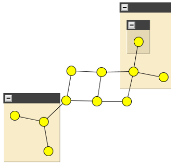
Рис. 24 – Вкладений граф.
