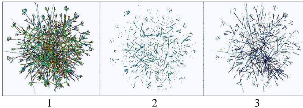
Рис. 1 – Структура мережі:
