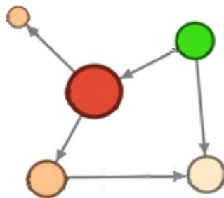
Рис. 33 – Результат розфарбування
